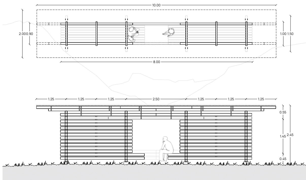
Plan et élévation nord de la cabane.
