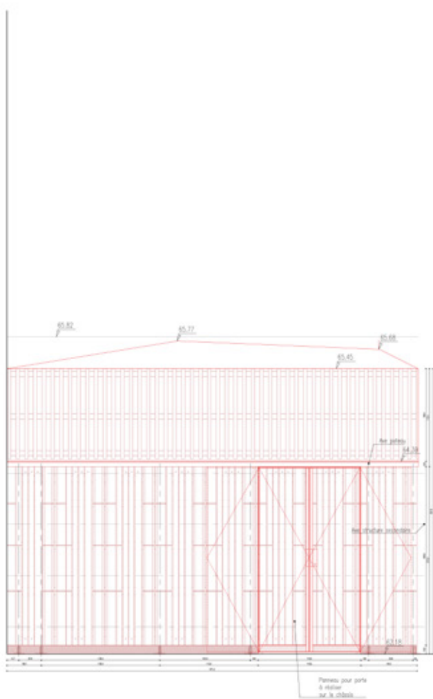
Façade ouest
