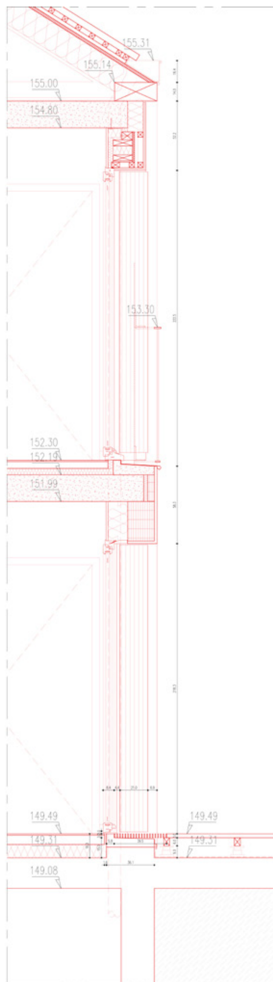
Coupes de détail d'enveloppe.
