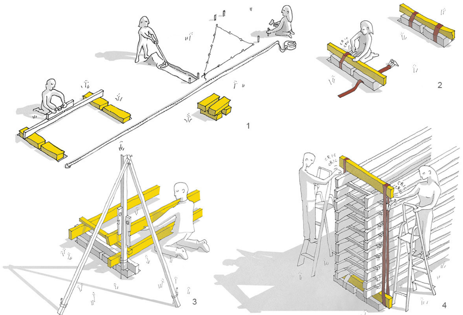
Montage de la cabane.
