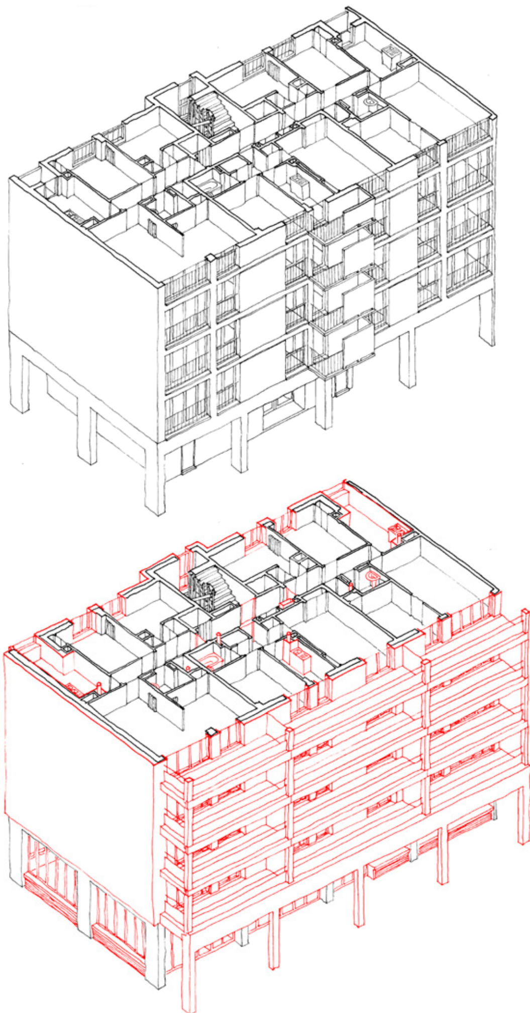
Extraits axonométriques d'une cage type existante et projetée.
